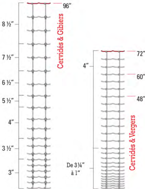
Clôture pour Cervidés & Vergers avec noeud Monarch®
